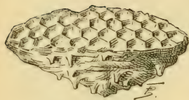
Fig. 32. — Michelinia favosca .
